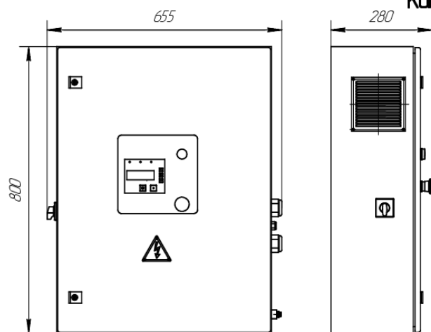
Блок управления
